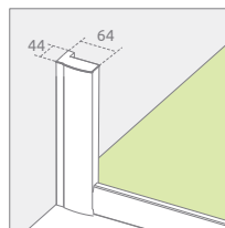
fali profil (ajtó) Premium Plus DWJ, DWJ+S, DWD
