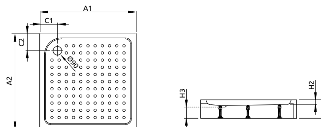
RODOS C zuhanytálca lábbal és ST 90 szifonnal
