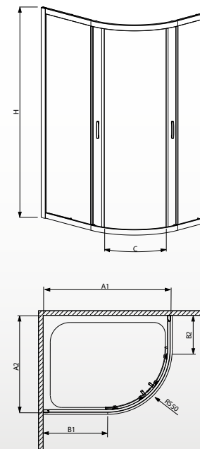
A kabin univerzális (fordítható).
