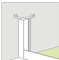
fali profil (ajtó) Treviso DW, DW+S
