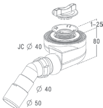
ST 90 zuhanytálca szifon, Ø90
