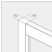
fali profil Twist DW+S
