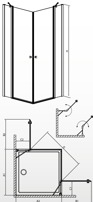
EOS II PDD 80B + PDD 80J = PDD 80x80 zuhanykabin.
