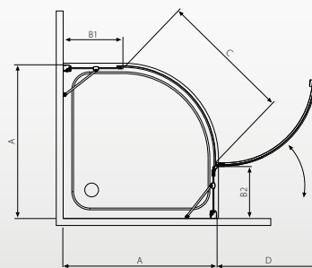
A rajzon balos zuhanykabin látható.
