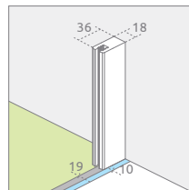
fali profil az oldalfalra Twist DW+S
