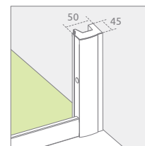
mágneses fali profil Premium Plus DWJ, DWJ+S
