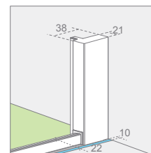
mágneses fali profil
