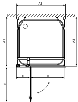
A rajzon balos zuhanykabin látható.
