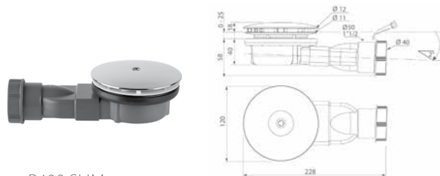
R400 SLIM zuhanytálca szifon, Ø90
