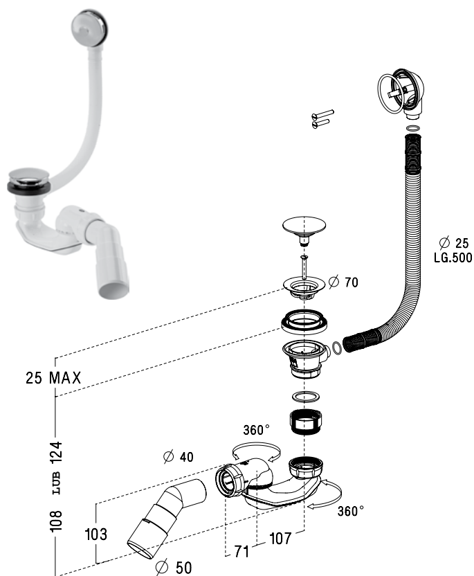
B602R zuhanytálca szifon, Ø70
