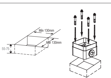
R-box
